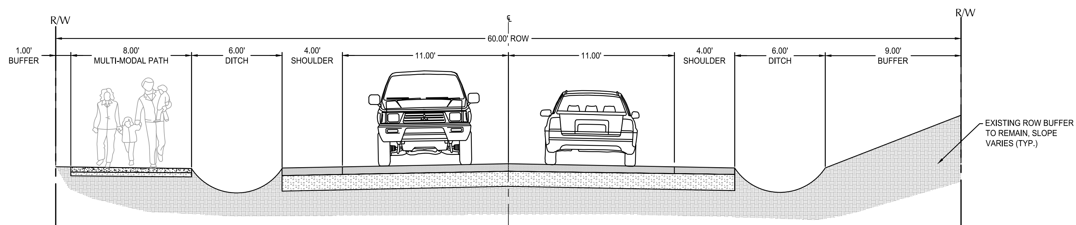
OPTION 1 SECTION SCALE: 1" = 4'
