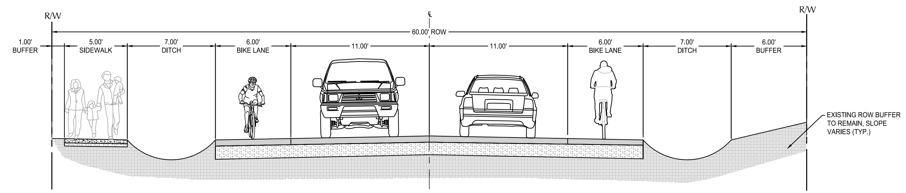
OPTION 2 SECTION SCALE: 1" = 4'
