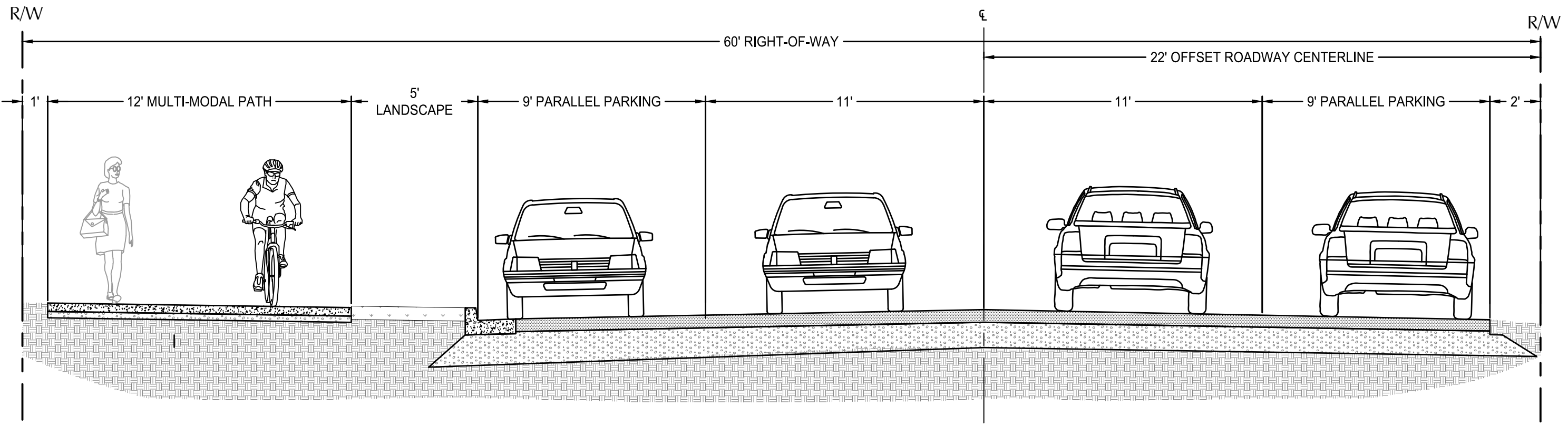
OPTION 3 SECTION SCALE: 1" = 4'
