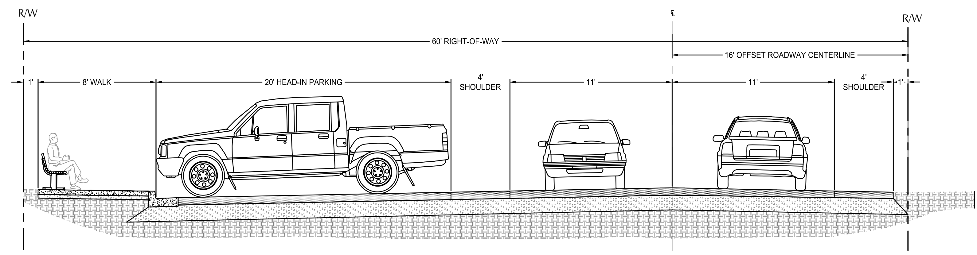
OPTION 1 SECTION SCALE: 1" = 4'
