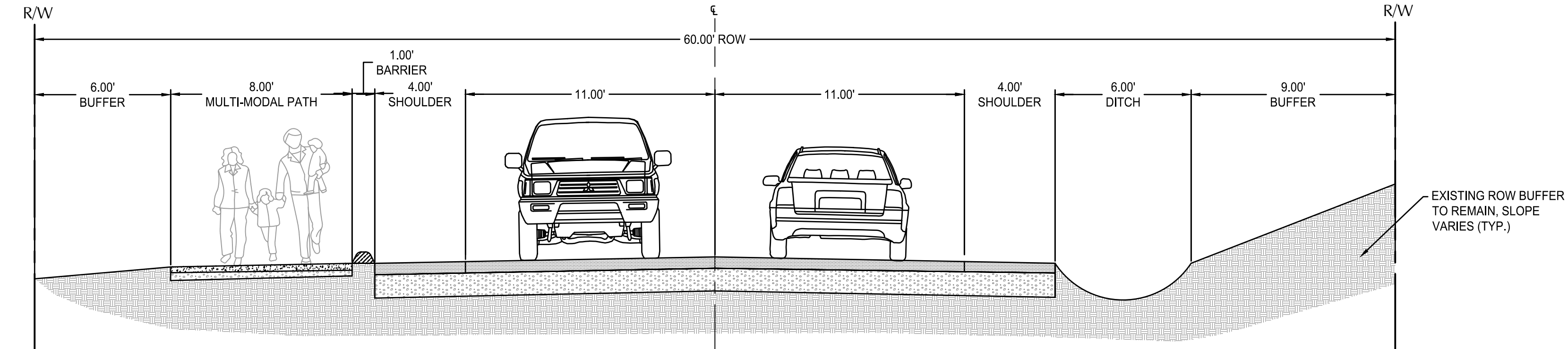
OPTION 3 SECTION SCALE: 1" = 4'
