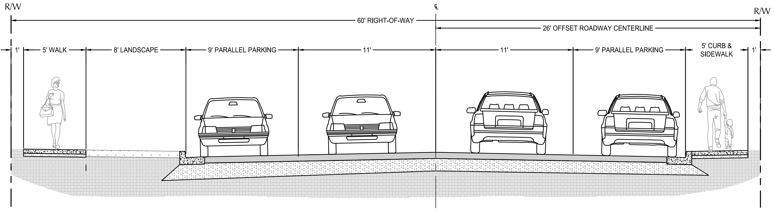
OPTION 2 SECTION SCALE: 1" = 4'
